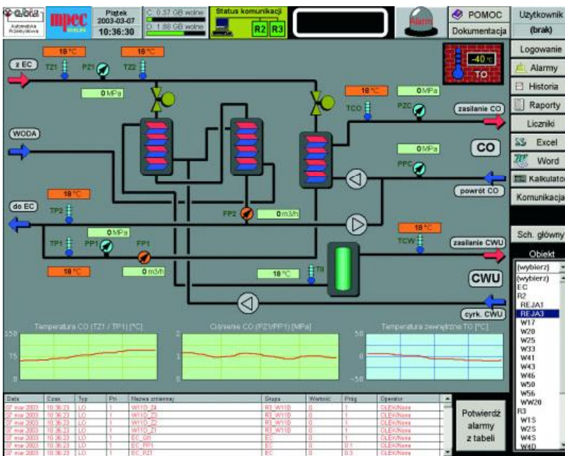
Rys. 3. Ekran technologii obiektu.
